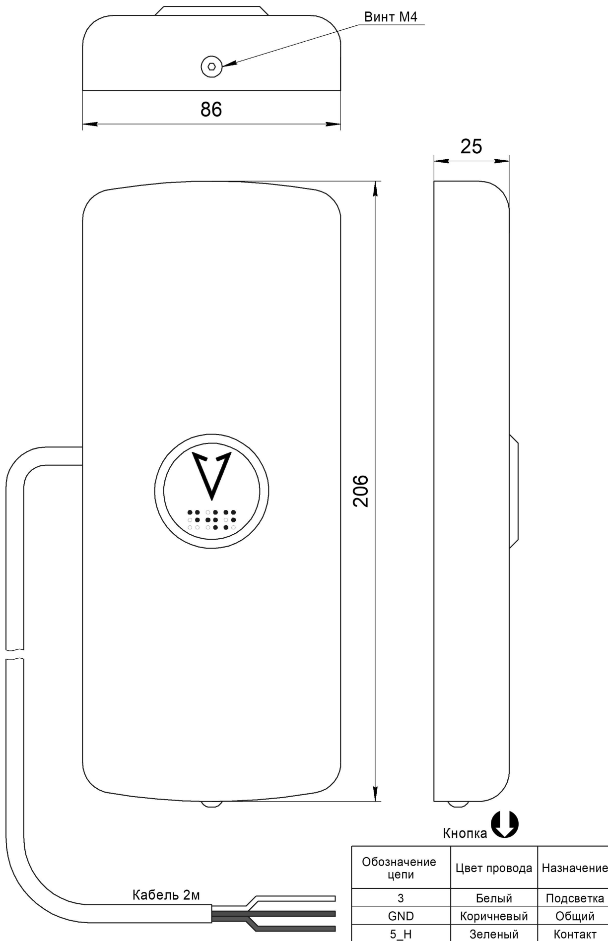
Рис.1 Внешний вид и габаритные размеры Вызывного поста ВП-1102-03
